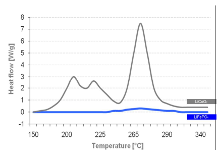
Thermische Stabilität der Fortelion Zelle in blau
